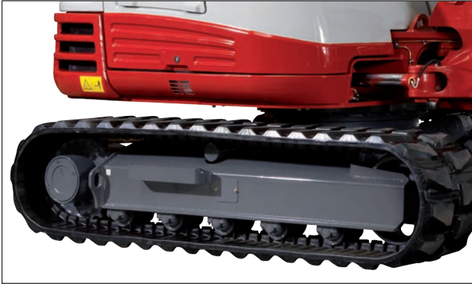
Rodillos con guía interior y exterior para un funcionamiento seguro de las cadenas de goma Double-Short- Pitch que evitan vibraciones durante la marcha.
